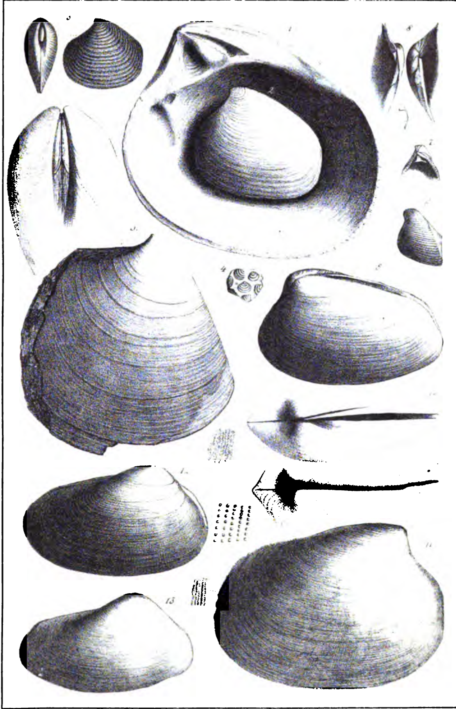
Auenstedt, Jura
